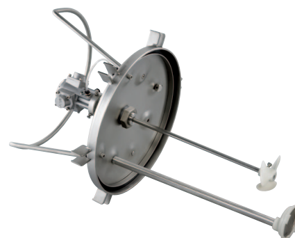
PNEUMATIC AGITATOR AM-6B
